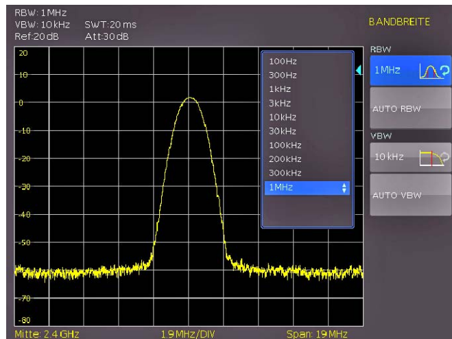
Abb. 6.2: Auswahlmöglichkeiten RBW
