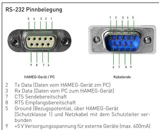
Abb. 12.1: Pinbelegung RS-232
