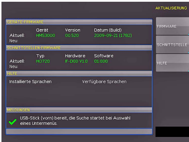
Abb. 9.2: Aktualisierungsmenü Firmware
