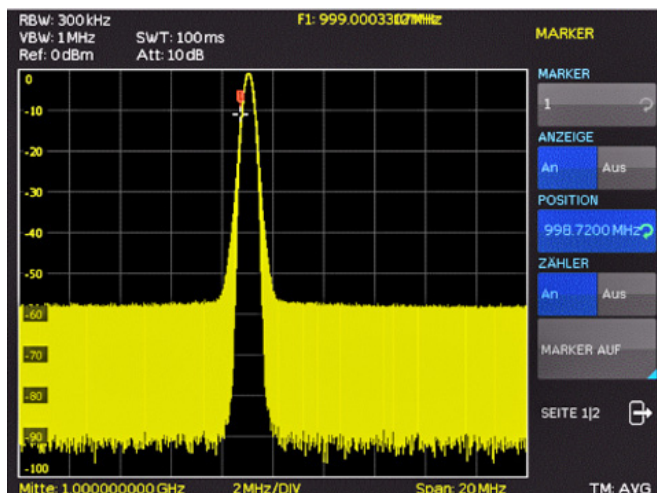
Abb. 6.7: Frequenzzähler
