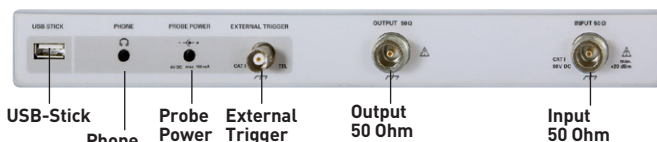
Abb. 10.1: Anschlüsse Geräte-Vorderseite
